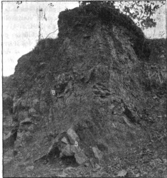
Fig. 1. Basalt und Schiefertons. Rechts von B (Basalt) der Ton. (Autor phot.)
